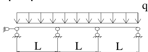
Допустимые расчетные снеговые нагрузки q , кгс/м 2
